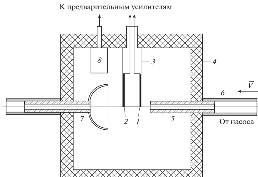
Рис. 2. Схема измерительной ячейки с электродами: 1, 2 — первый и второй электроды, 3 — диэлектрический цилиндр, 4 — корпус ячейки, 5 — инжектор, 6 — трубопровод, 7 — уловитель потока, 8 — опорный электрод.
