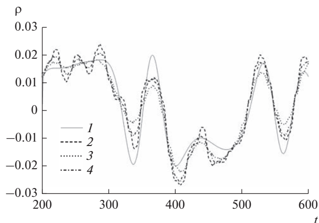
Рис. 2. Иллюстрация расшифрованной информации при наличии шумовых помех в канале связи: 1 – исходная информация; 2 – после получения сигнала из зашумленного канала связи с применением фильтра нижних частот; 3 – с применением медианного фильтра; 4 – после применения комбинированного фильтра.
