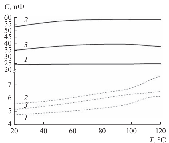
Рис. 7. Зависимость C_{\max} (сплошные линии) и C_{\min} (штриховые линии) МДП-структур от температуры для структур 1...3.
