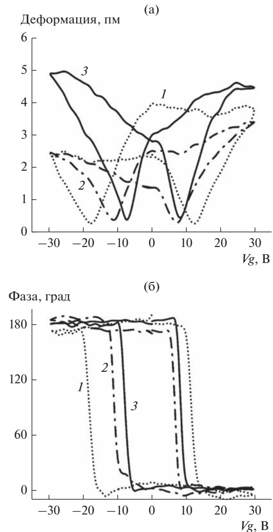
Рис. 3. Зависимость амплитуды (а) и фазы сигнала пьезоотклика (б) от постоянного напряжения для образцов 1...3.
