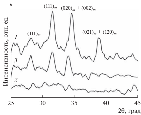
Рис. 1. Рентгеновская дифрактограмма пленок HfO 2 1...3.
